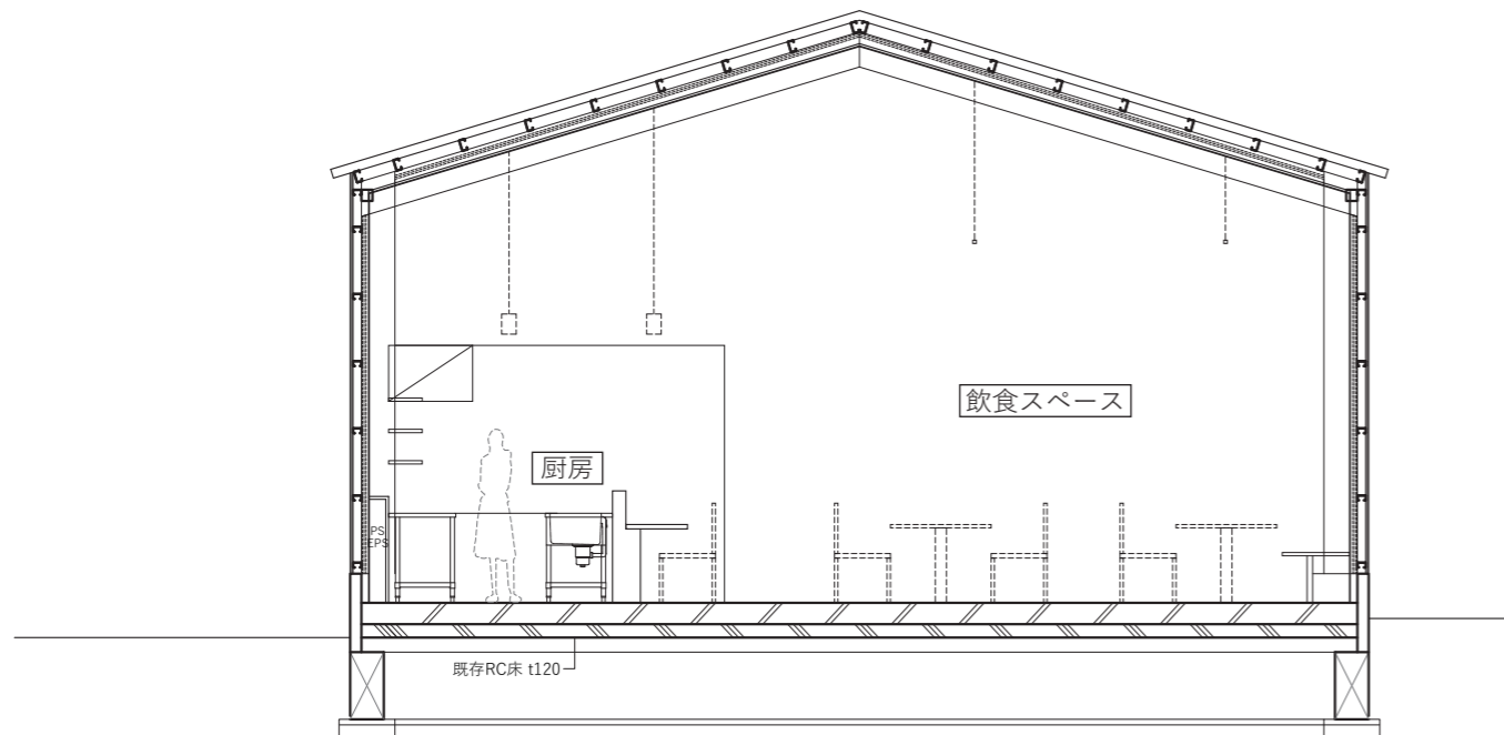
短手断面図 1
