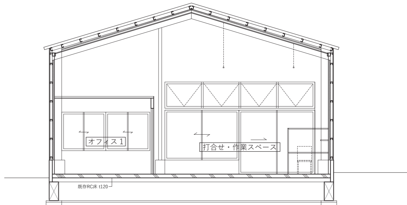
短手断面図 2
