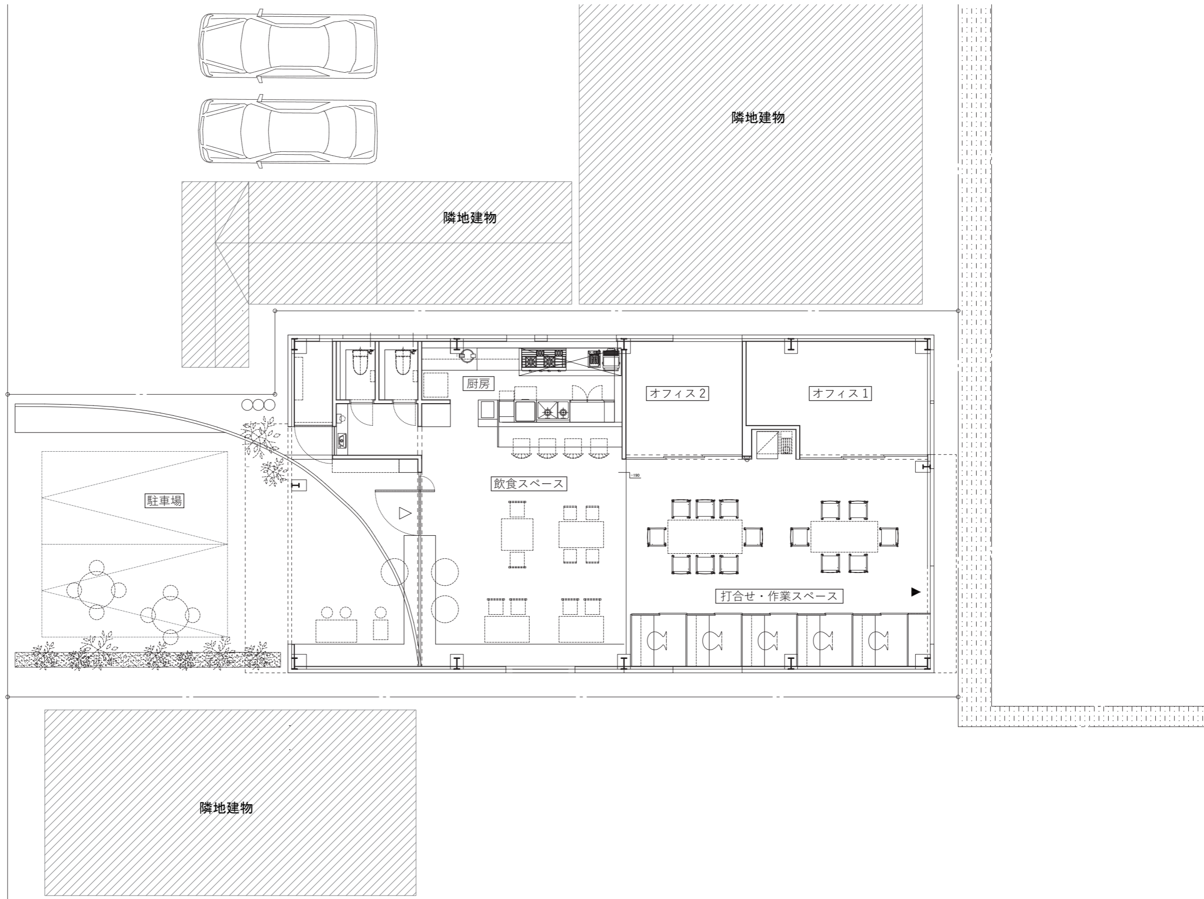
平面図
