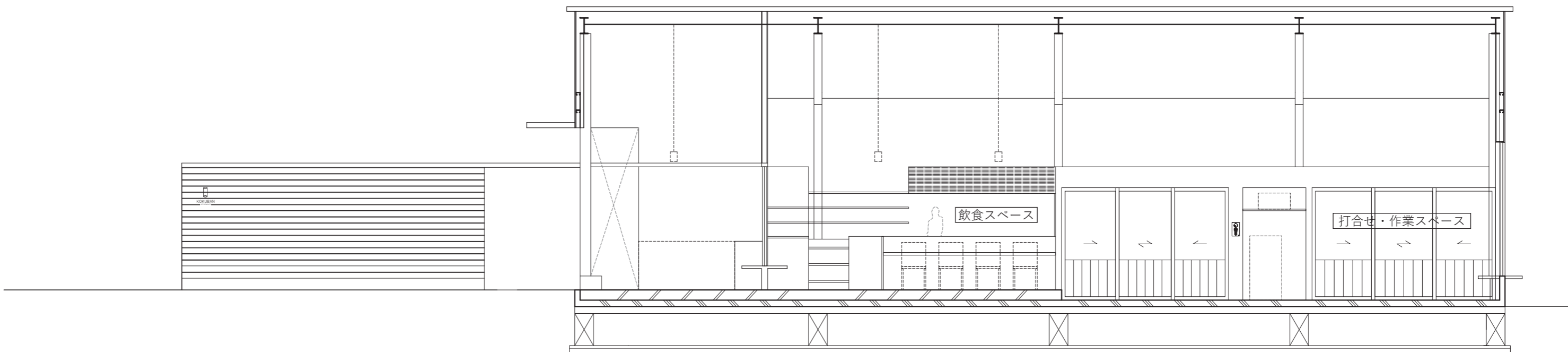
長手断面図
