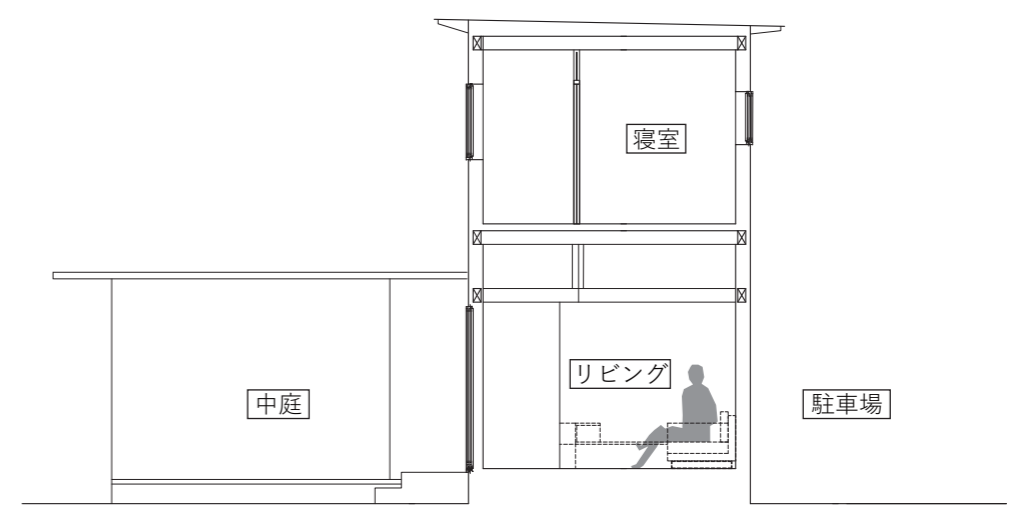
短手断面図
