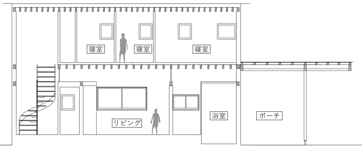
長手断面図
