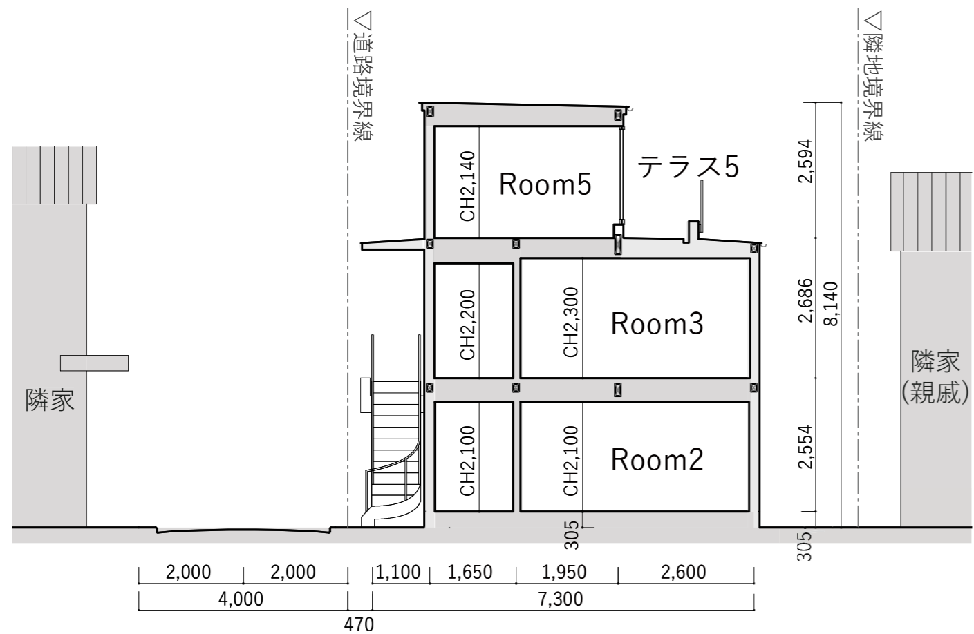
東西断面図
