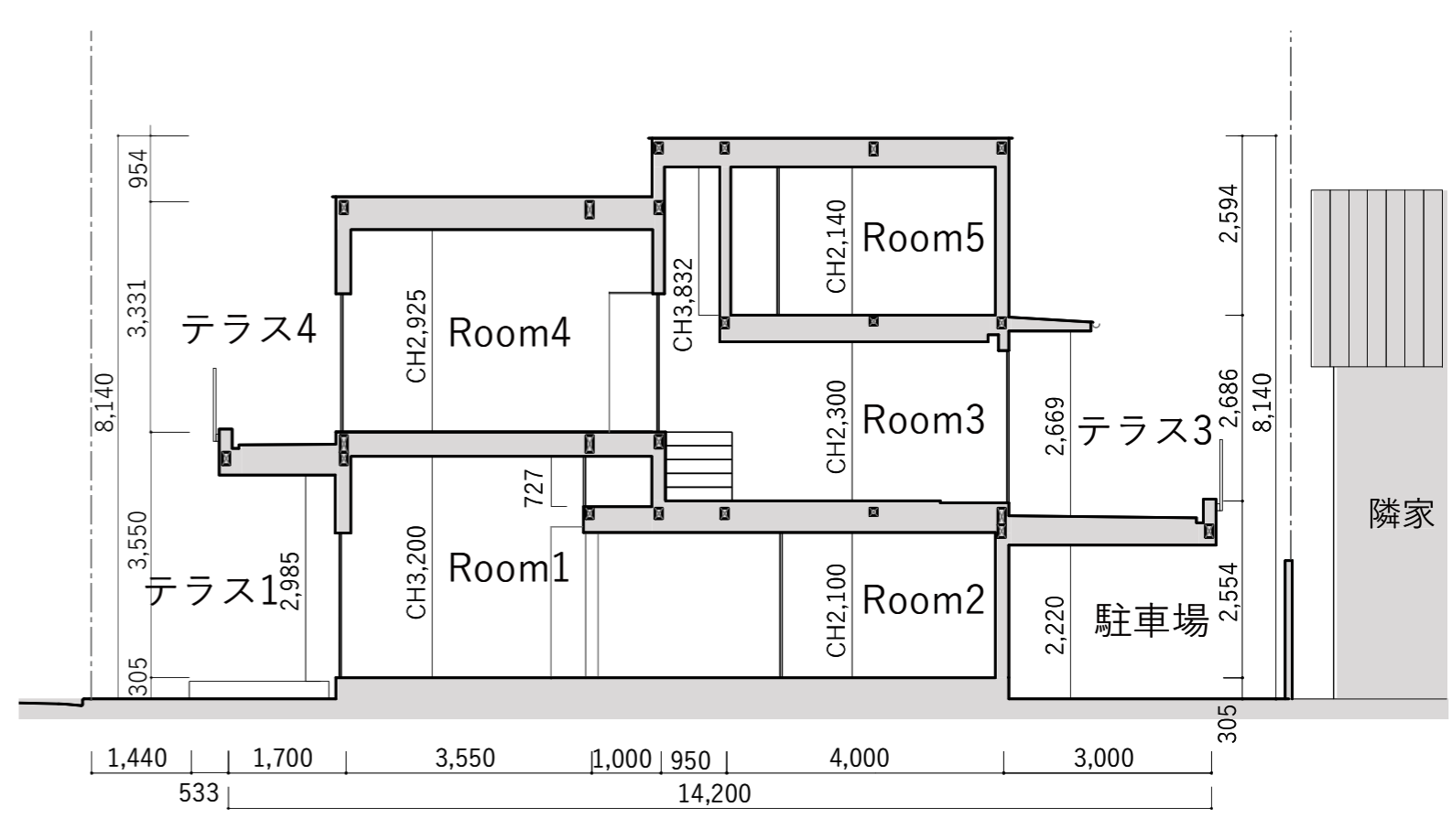
南北断面図
