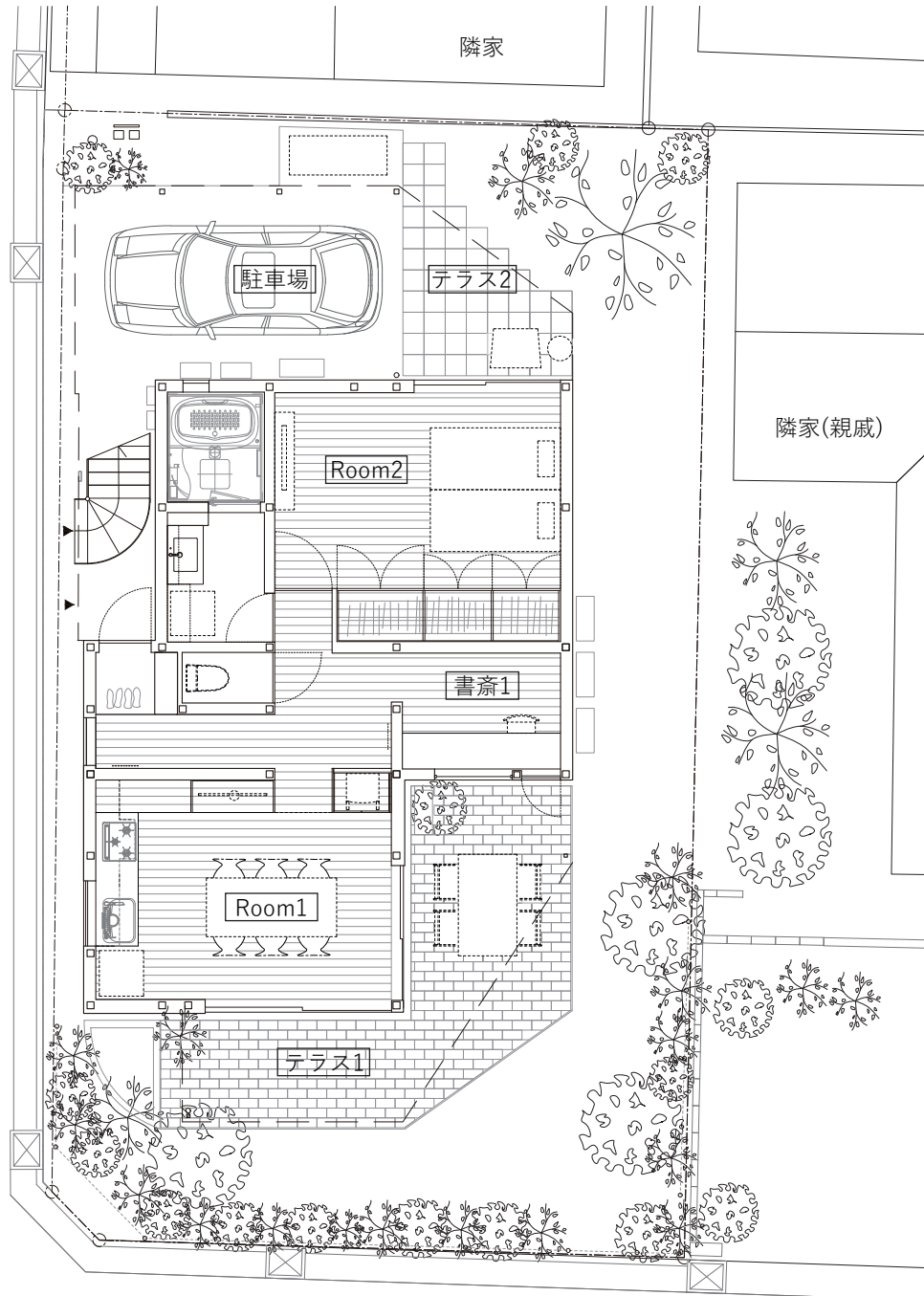
1階平面図
