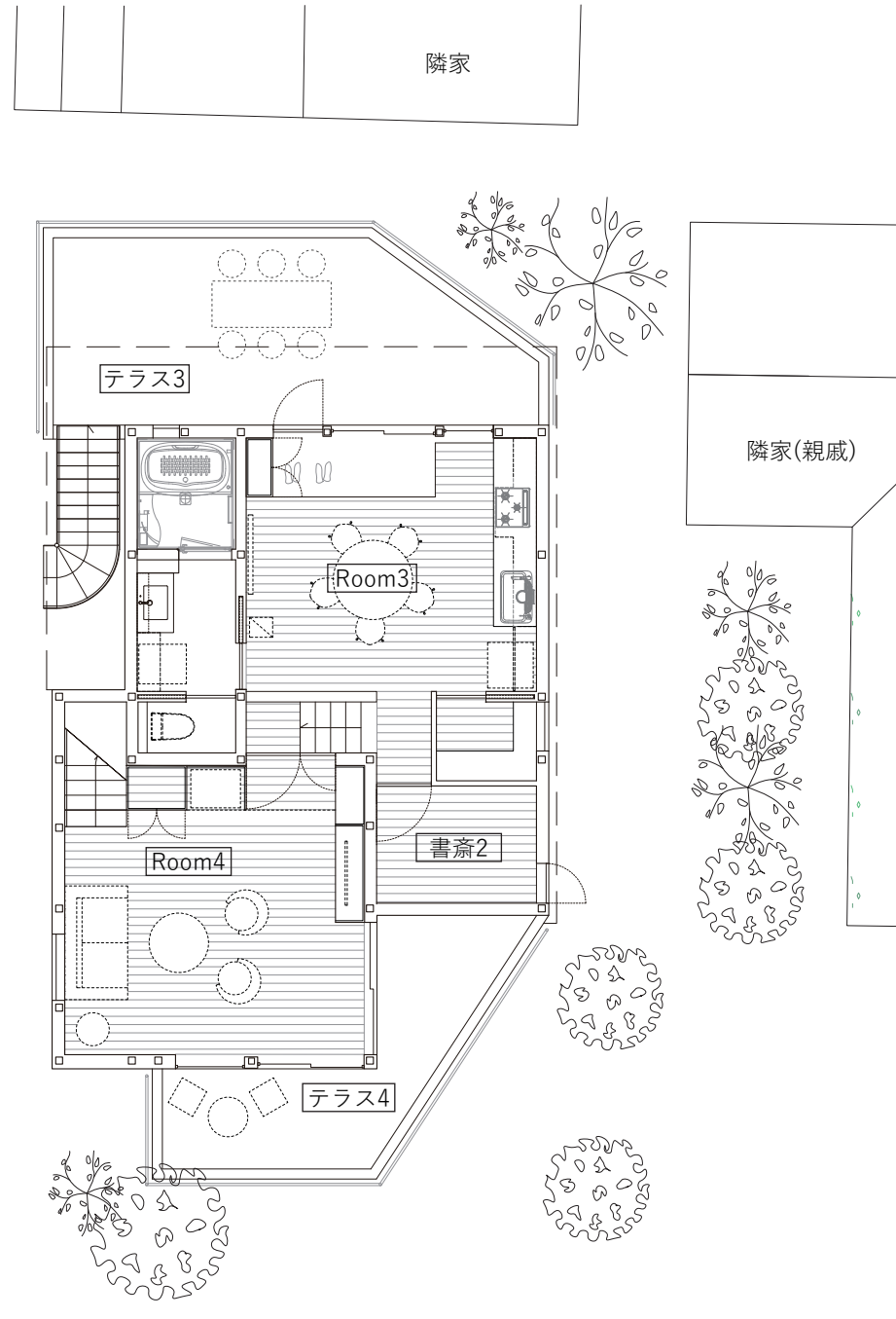
2階平面図
