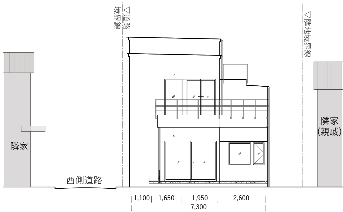
南立面図
