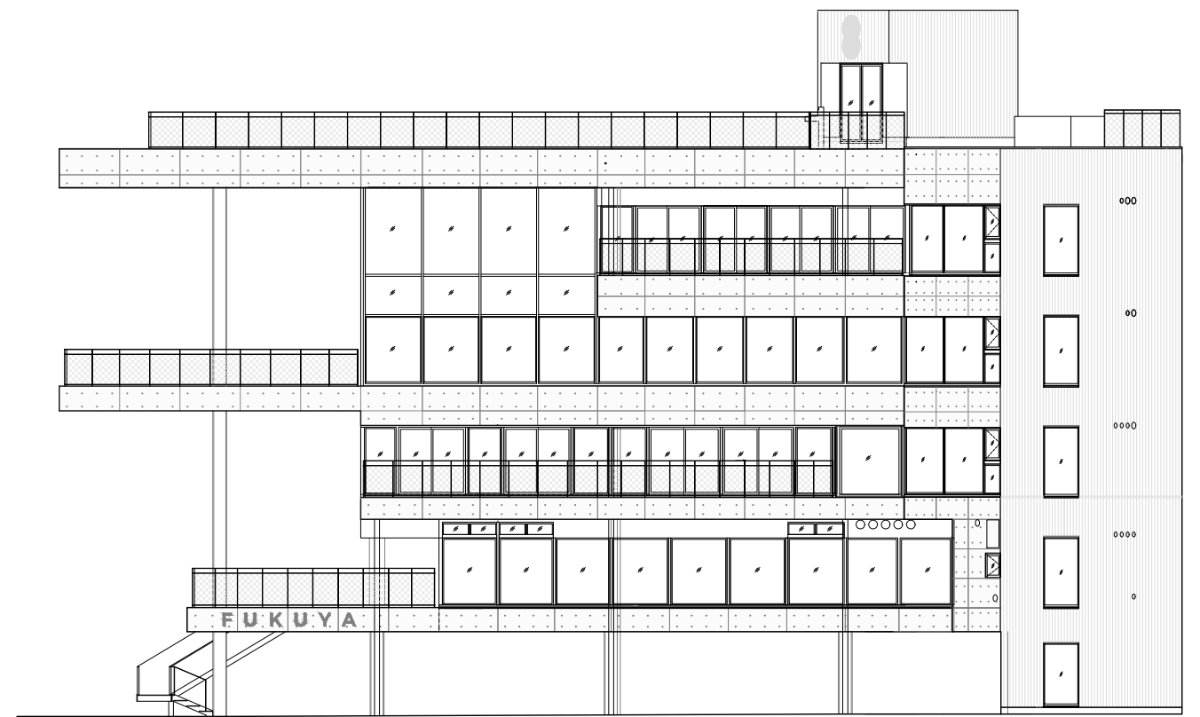
南東立面図
