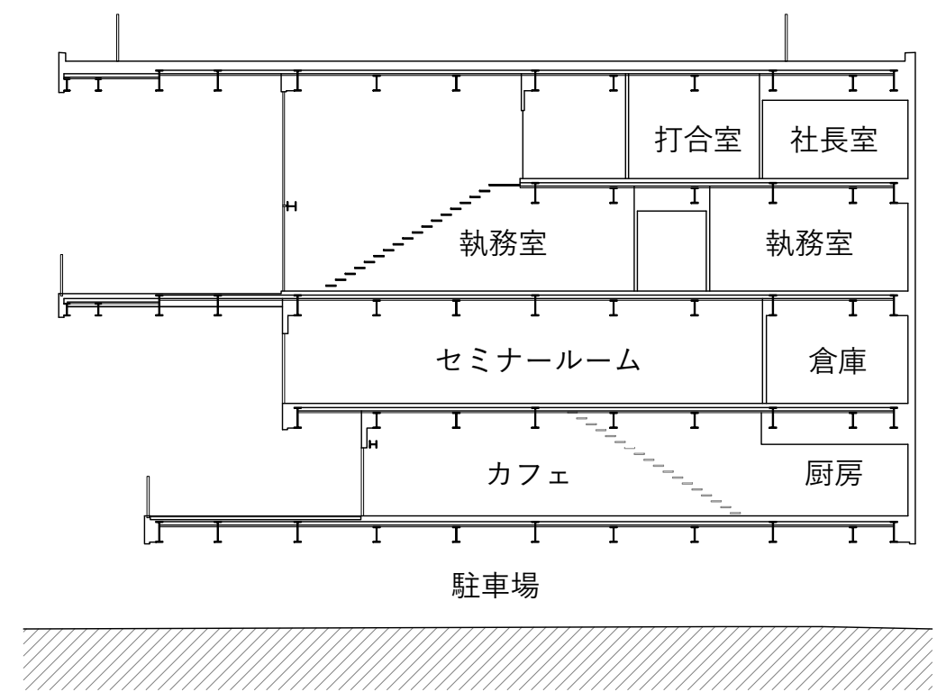
南北断面図
