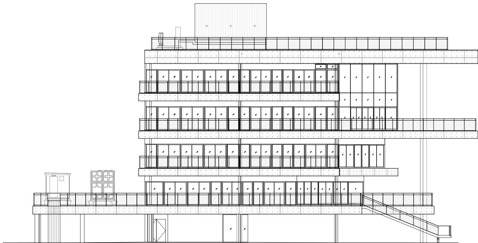
西立面図
